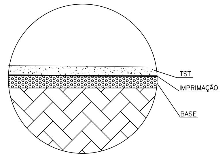
DET. CAMADA DE TST
