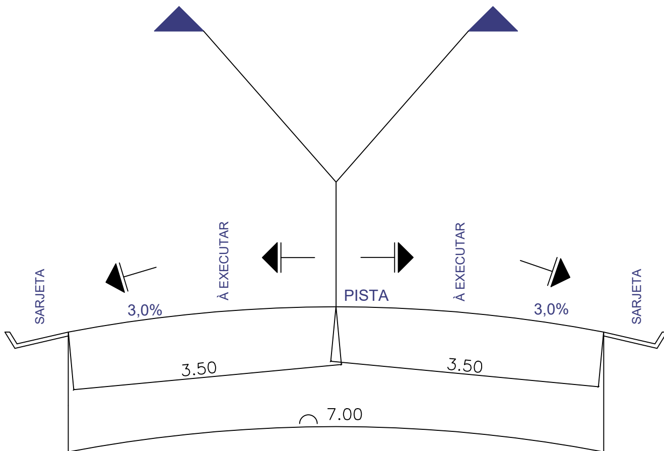
DET. GENÉRICO 2 - DUAS SARJETAS
