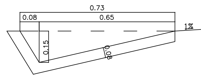
DET. SARJETA TRIANGULAR
