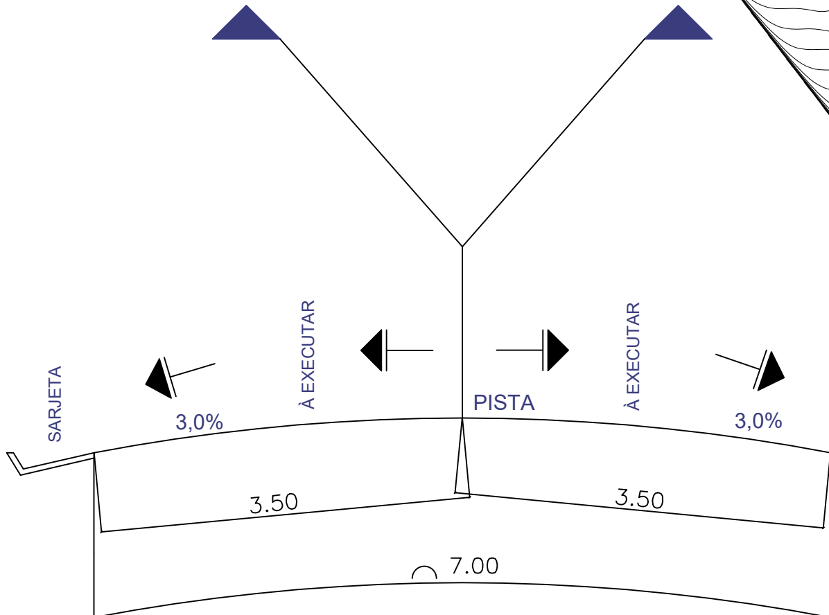
DET. GENÉRICO 1 - UMA SARJETA
